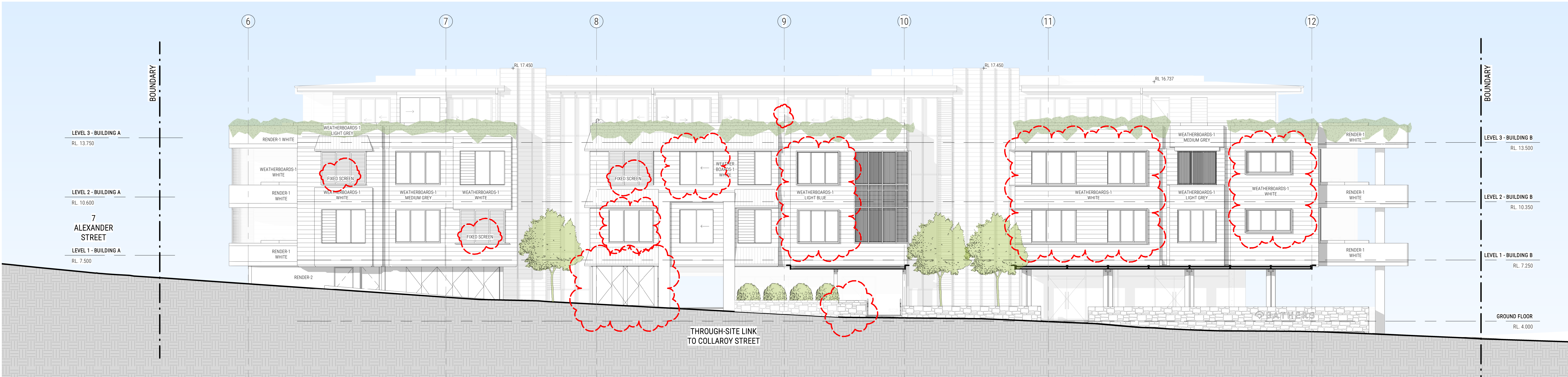
2 SOUTHERN ELEVATION - DA DA010 1:100 @ A1
